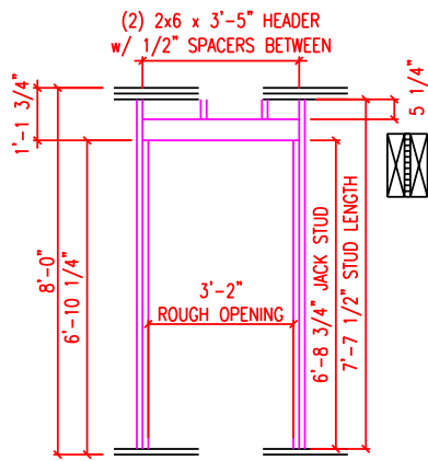
EXTERIOR DOOR FRAMING
